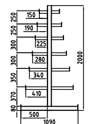
Draagarm dubbel
