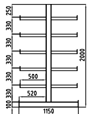
Draagarm dubbel
